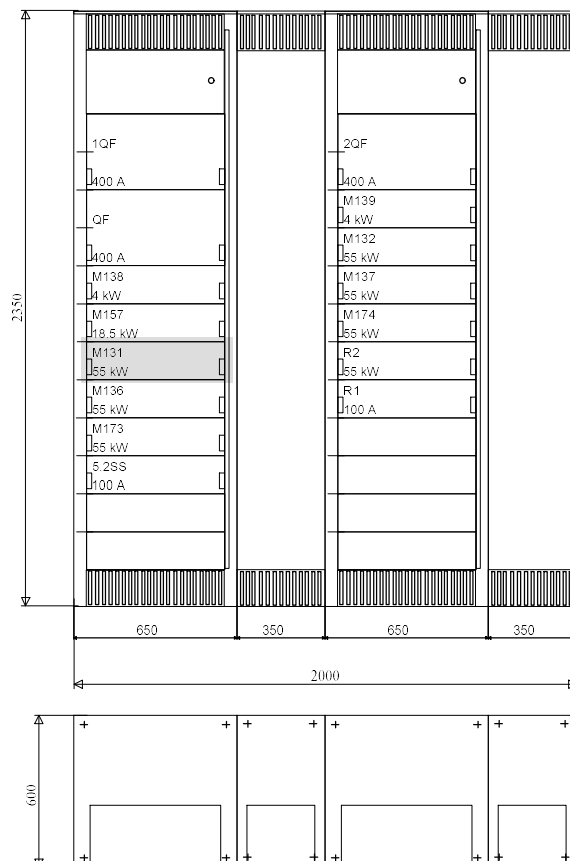
Рис. 10.2. Внешний вид распределительного щита в конструктиве Systeme Gear (пример) по однолинейной схеме на рис. 10.1.
